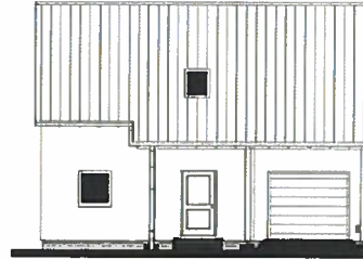
POHLED SEVERNÍ
